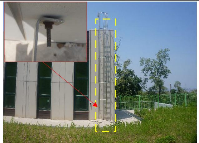
건축구조물 옥상층 진입사다리 볼트이완
