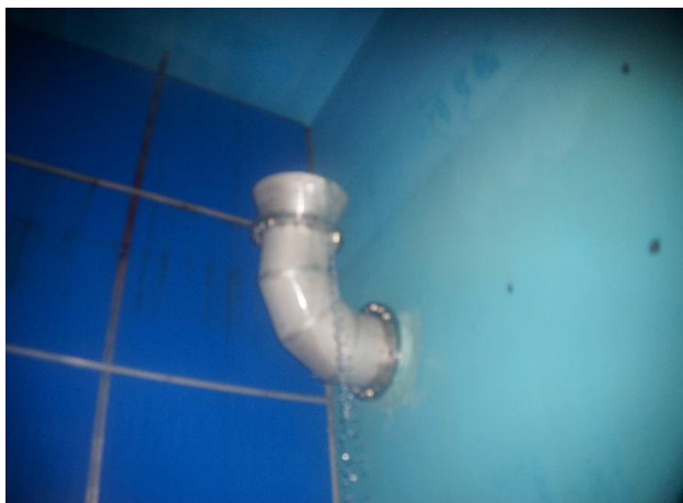
배수지 1지 유입관 상태양호
